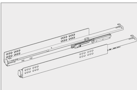
Plnovýsuv Quadro V6 Nosnost 30 kg ► se Silent System nebo Push to open
