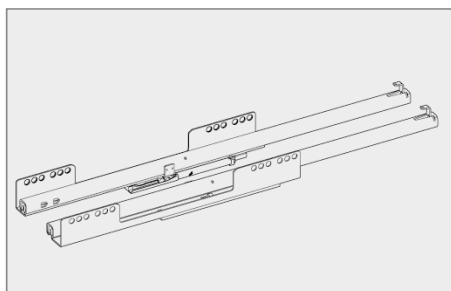
Částečný výsuv Quadro 25 Nosnost 25 kg ► se Stop Control nebo Silent System
