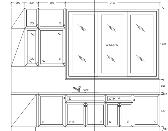
ELEVATION 'C'
