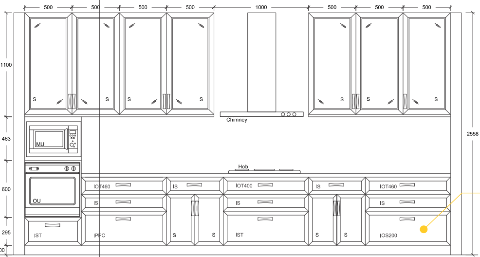
ELEVATION 'B'
