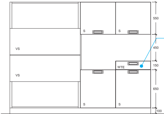
ELEVATION 'B'
