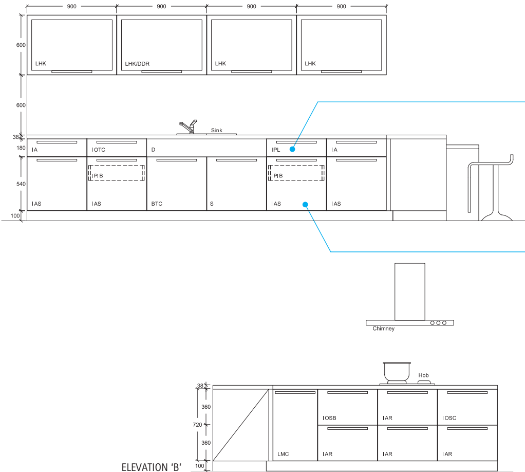
ELEVATION 'B'
