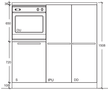
ELEVATION 'B'
