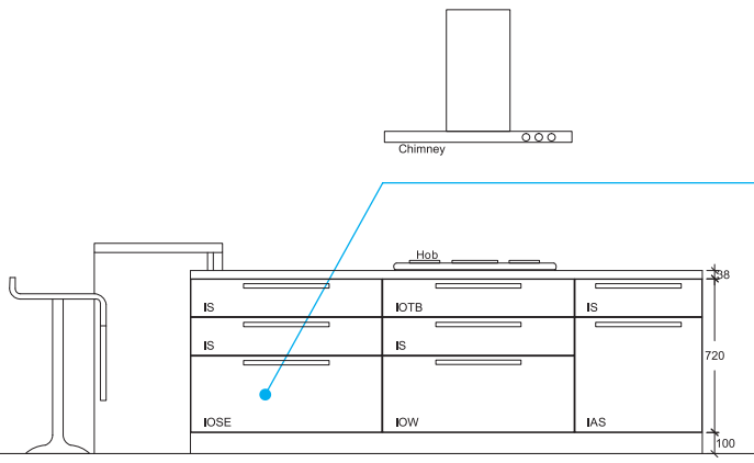
ELEVATION 'C'
