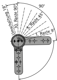
FrankoFlex Nullstellung 90°
